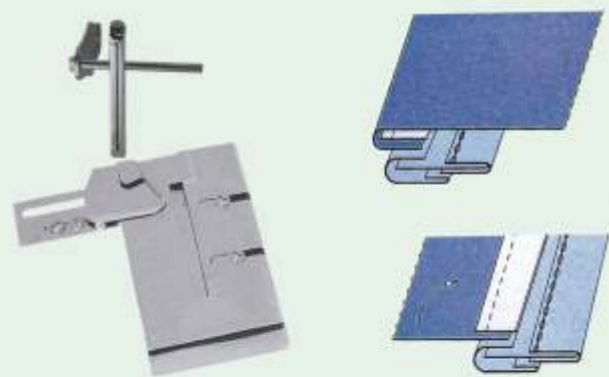
JZ-15570 单针袋口折边器
